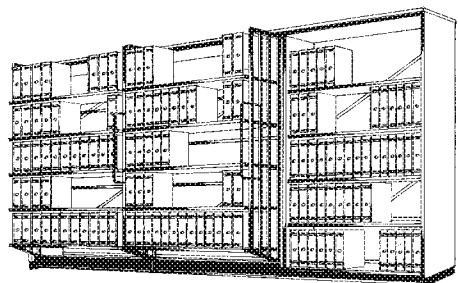
Vorsatzgleitregalanlage OGR/5-.../55
